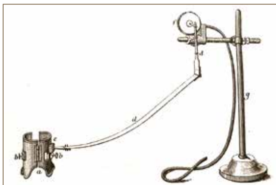
Рефлексограф для записи коленных рефлексов, предложенный В.М. Бехтеревым
